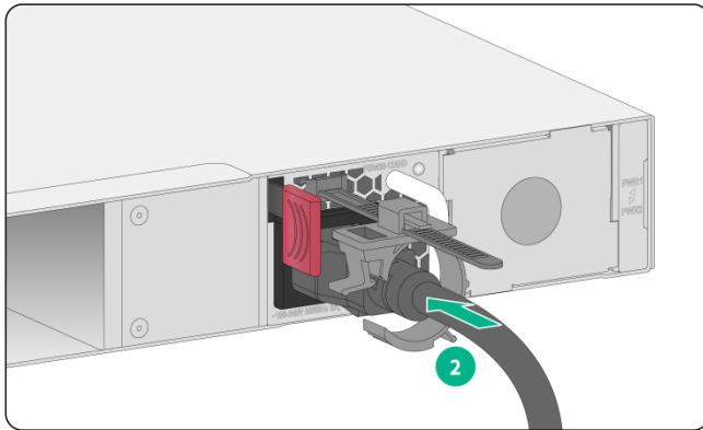
图2-27 PSR450-12AHD 电源模块电源线连接示意图三
