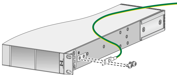
图2-8 安装接双孔端子接地电缆到主接地点的示意图
