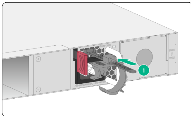
图2-25 PSR450-12AHD 电源模块电源线连接示意图一
