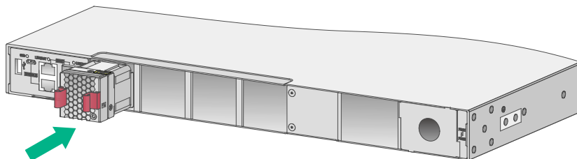
图2-14 风扇模块安装示意图
