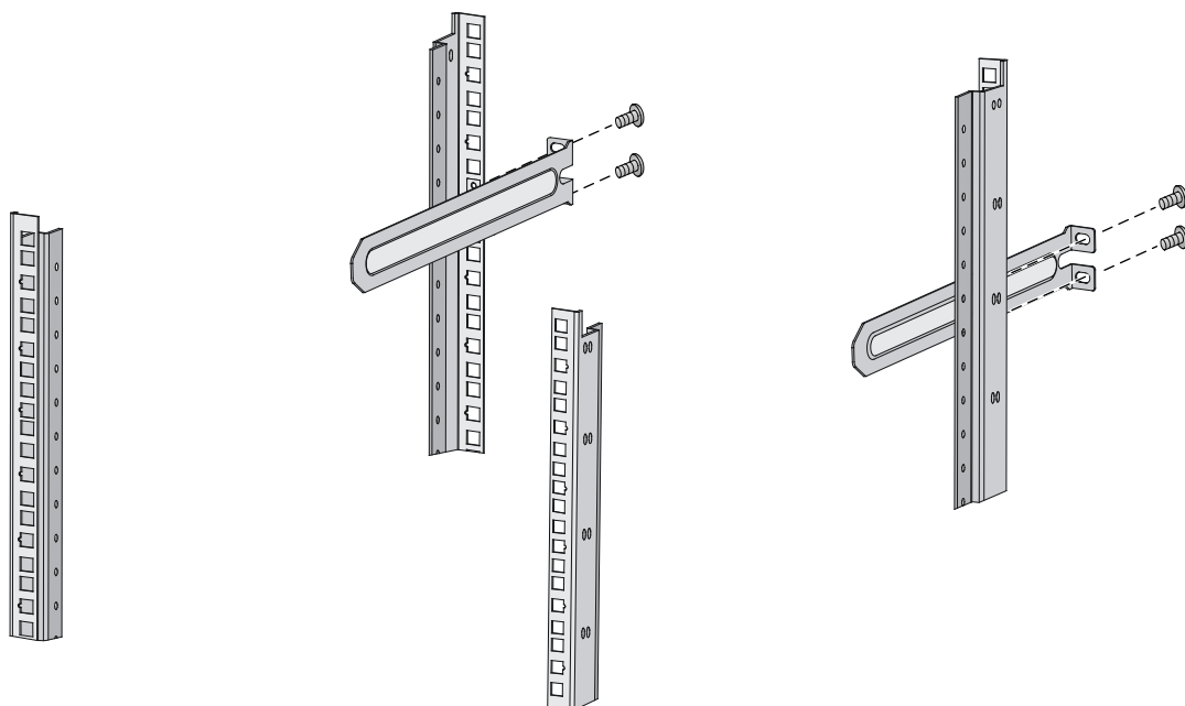
图2-9 滑道安装示意图
