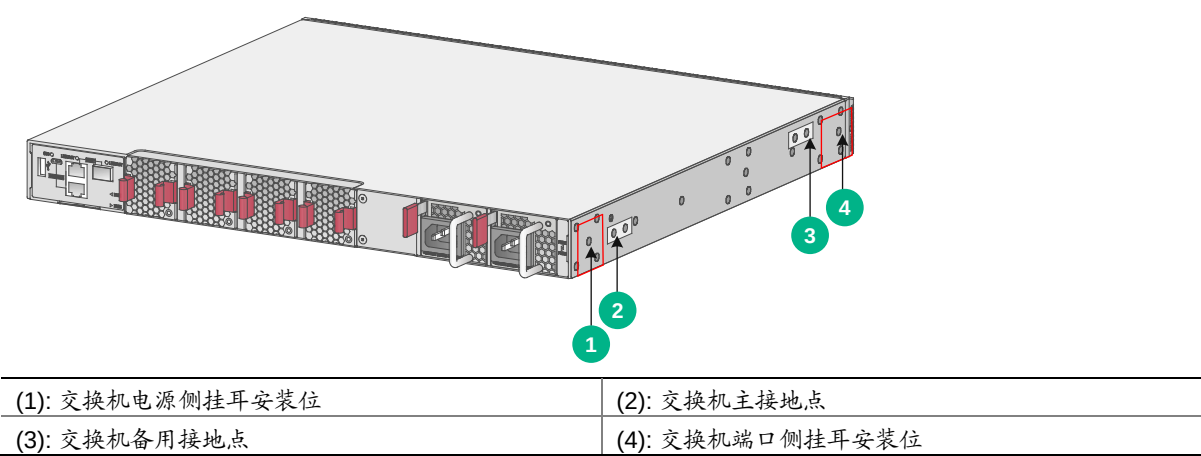
图2-5 S6600XP-54XG-EI-G 挂耳安装位置、接地线缆连接位置
