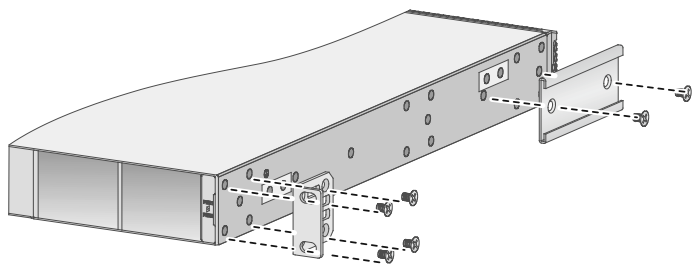
图2-6 安装挂耳和滑道导轨到机箱的示意图
