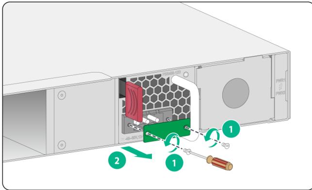
图2-29 PSR450-12D 电源模块电源线连接示意图二
