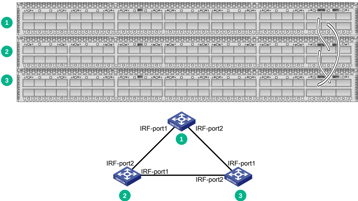
图4-3 IRF 环型连接方式及对应的拓扑示意图
