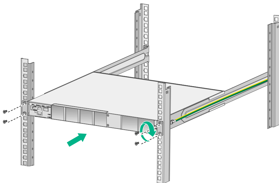
图2-10 安装交换机到机柜示意图（挂耳安装在靠近电源侧）
