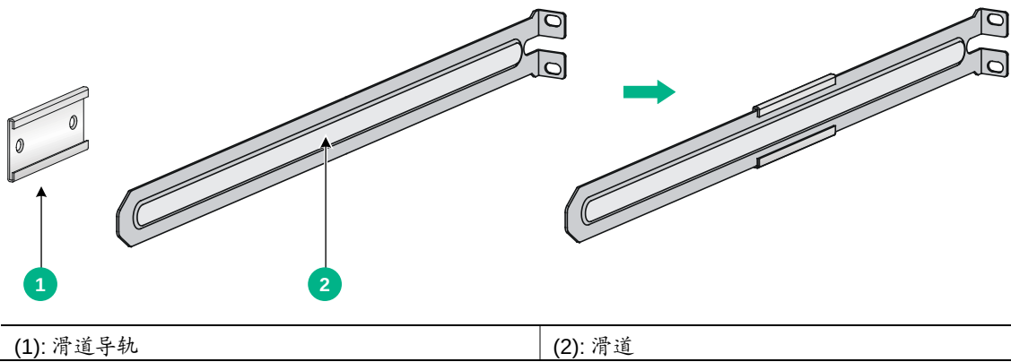
图2-3 1U 滑道及滑道导轨示意图
