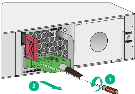
图2-23 拆卸 PSR450-12D 电源模块
