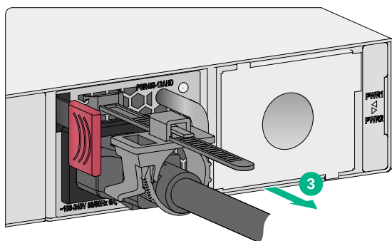
图2-22 拆卸 PSR450-12AHD 电源模块一
