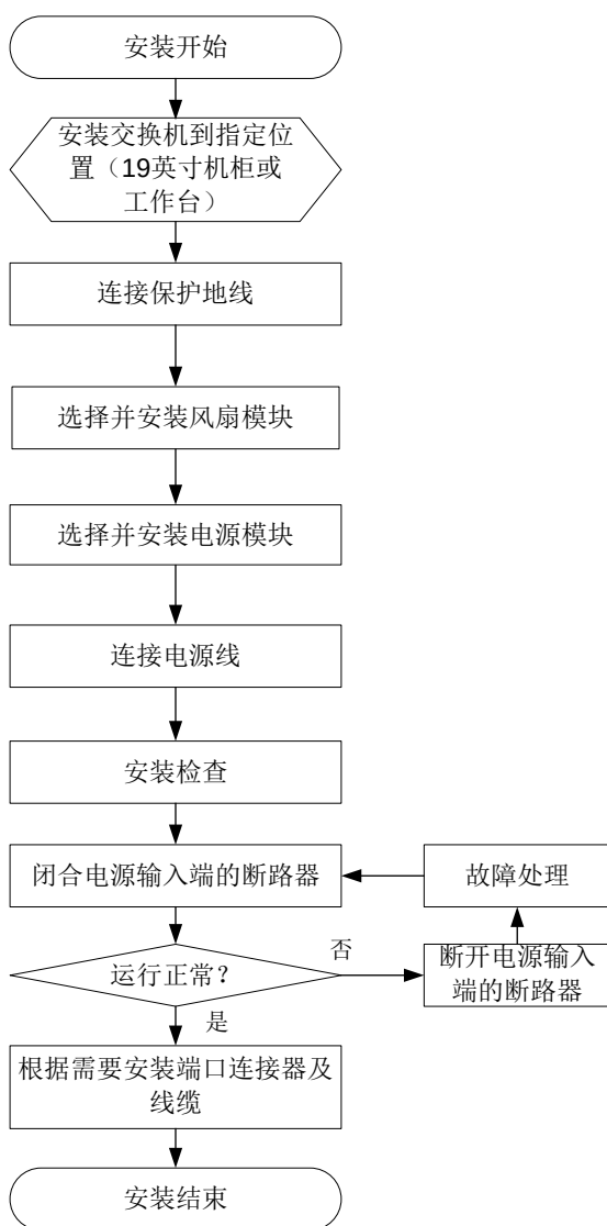
图2-1 交换机安装流程
