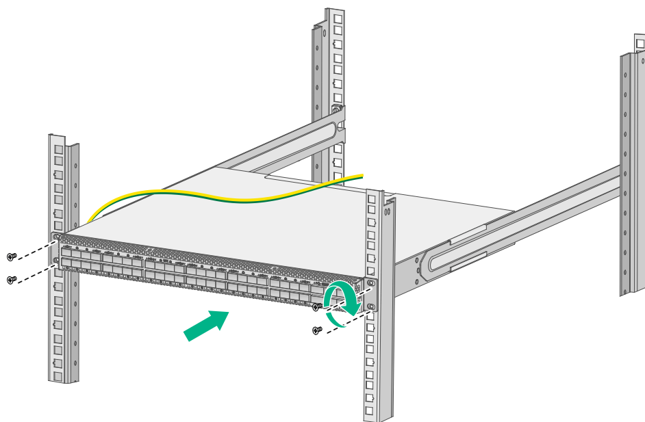
图2-11 安装交换机到机柜示意图（挂耳安装在靠近端口侧）
