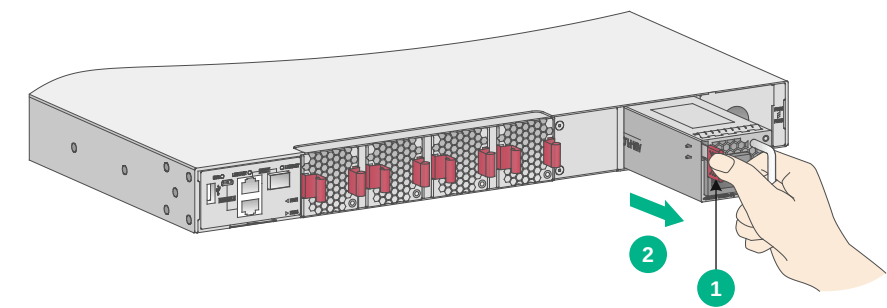
图2-20 拆卸 PSR250-12A/PSR250-12A1/PSR450-12A1 电源模块示意图
