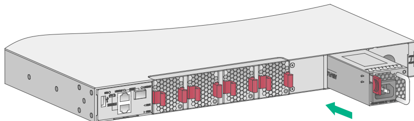
图2-18 电源模块安装示意图
