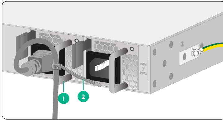
图2-24 PSR250-12A/PSR250-12A1/PSR450-12A1 电源线连接示意图
