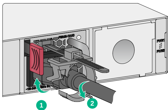
图2-21 拆卸 PSR450-12AHD 电源模块一
