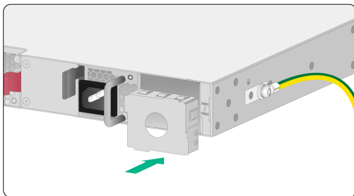
图2-19 电源假面板安装示意图
