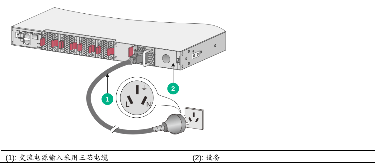
图2-13 利用交流 PE 线接地时接地安装示意图
