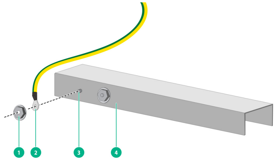
图2-12 连接接地线缆到接地排
